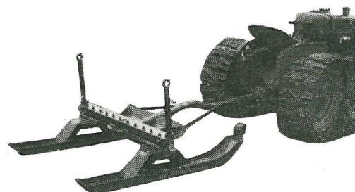
Lunningskälke ÖSA-18 (För Helbands-, Halvbands- och Hjultraktorer)
