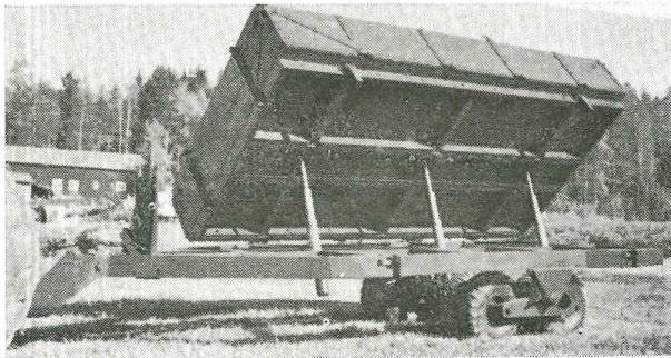
Flak med tipp för ÖSA-28
