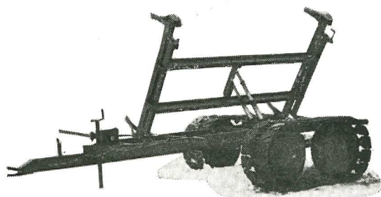
Bandvagn ÖSA-56
