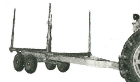
Traktorsläpvagn ÖSA-20-Timmerboggie
