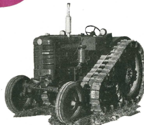
Halvbandsutrustningen ALFTA ÖSA-55 B
