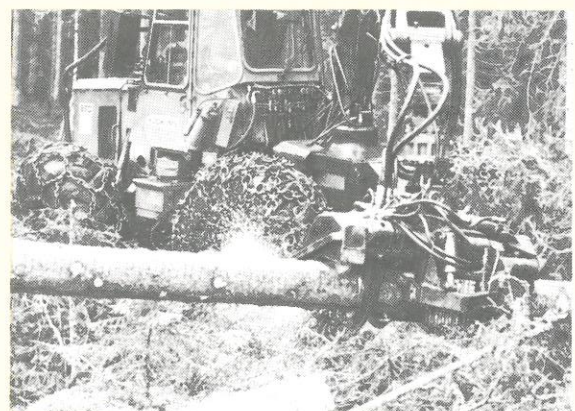
ÖSA 756 – effektiv engreppsskördare i slutavverkning.
