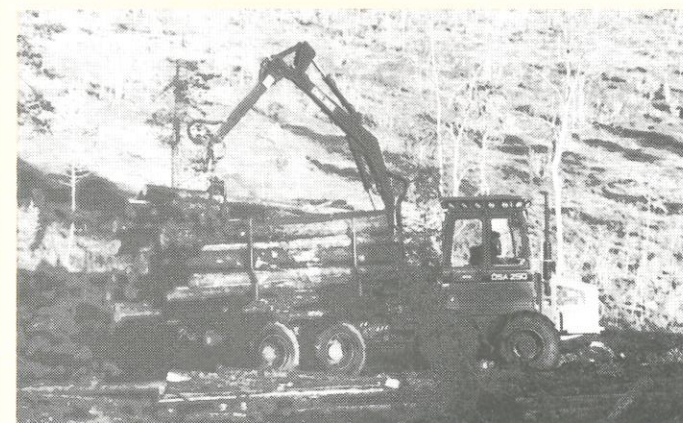
ÖSA 250 – en 10 tons skotare som är morgondagens basmaskin idag – enkel i uppbyggnad – mångsidig i användning.
